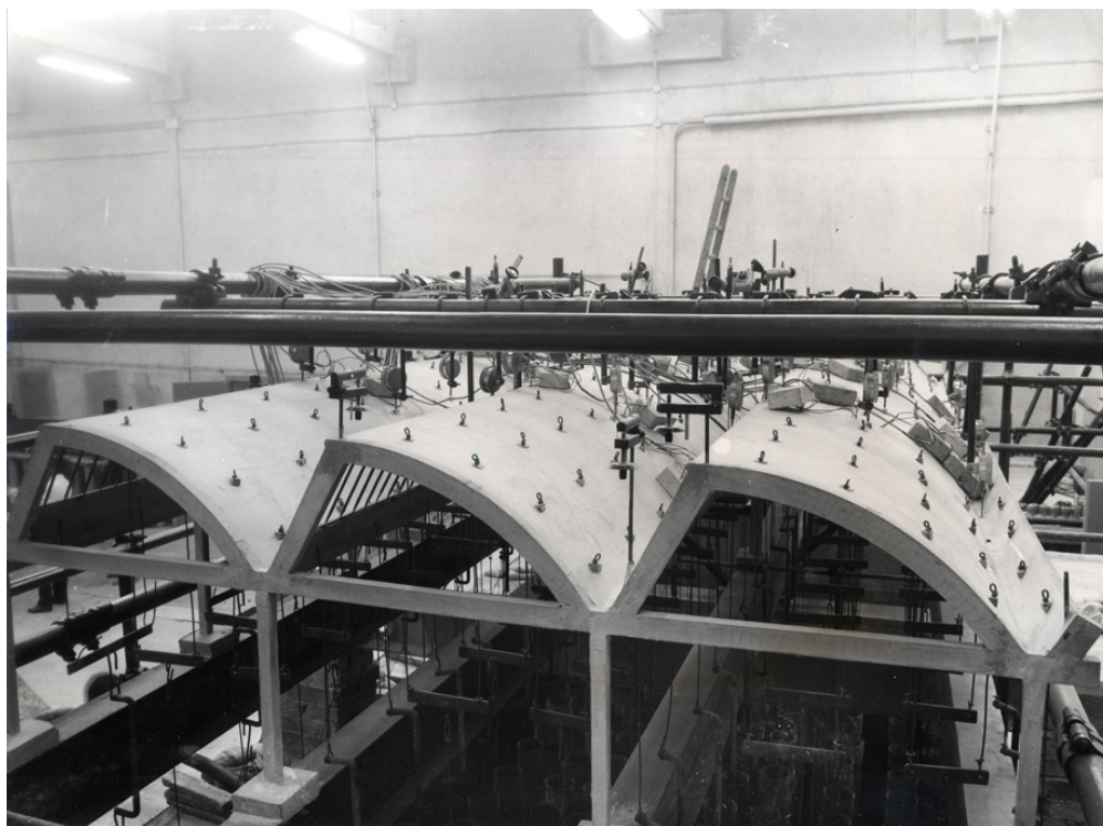
Vista de modelo reducido
