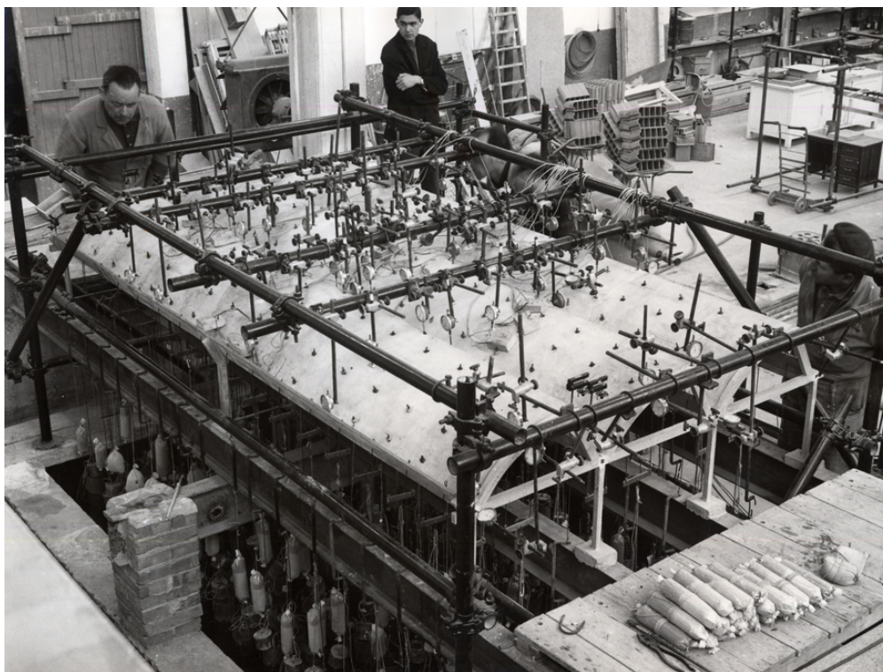
Vista de modelo reducido y técnicos
