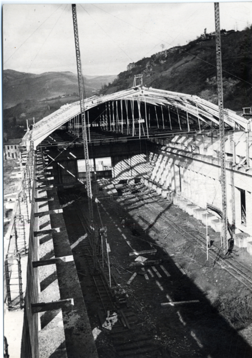
Vista interior de la factoría en construcción
