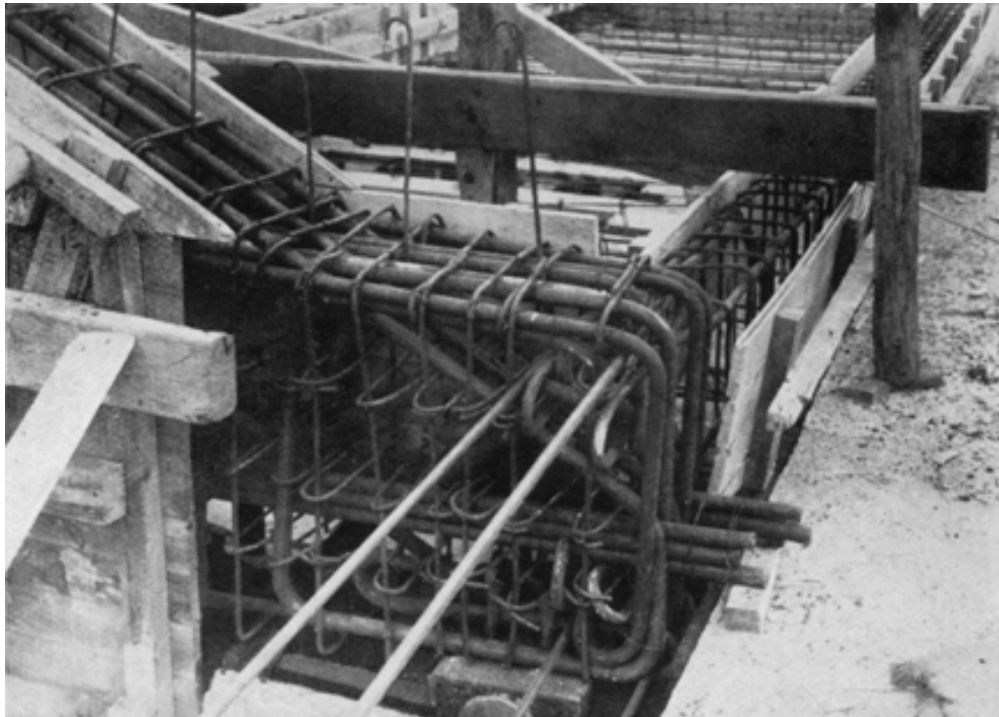
Detalle de construcción
