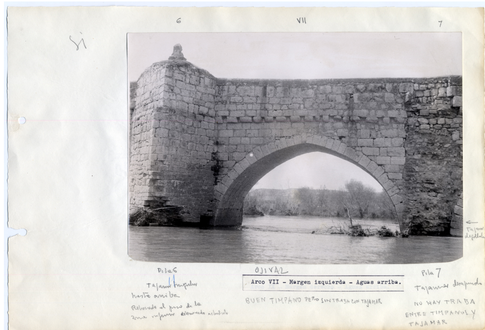
Detalle del puente
