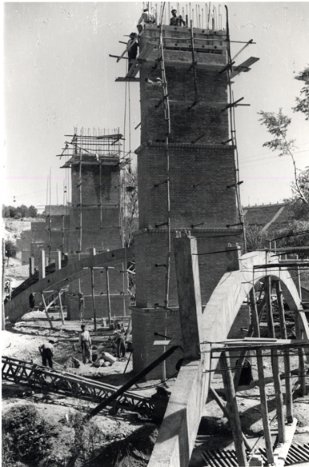
Detalle de la construcción de los pilares
