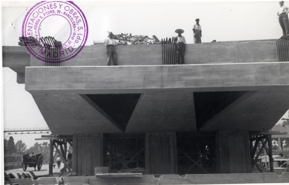
Detalle del puente en construcción
