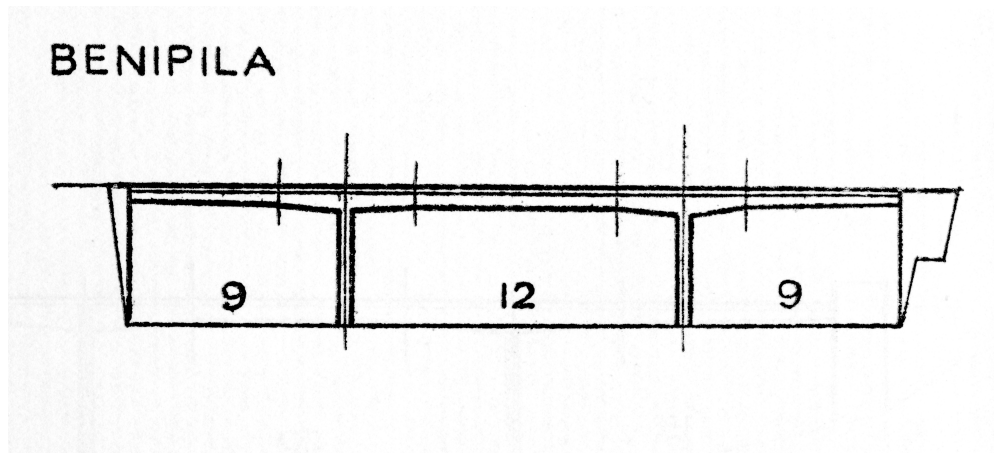
Alzado del puente con medidas de los vanos
