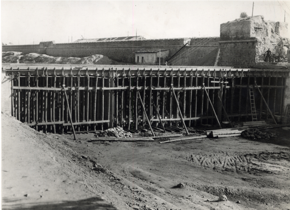
Cimbra de madera durante el proceso de construcción
