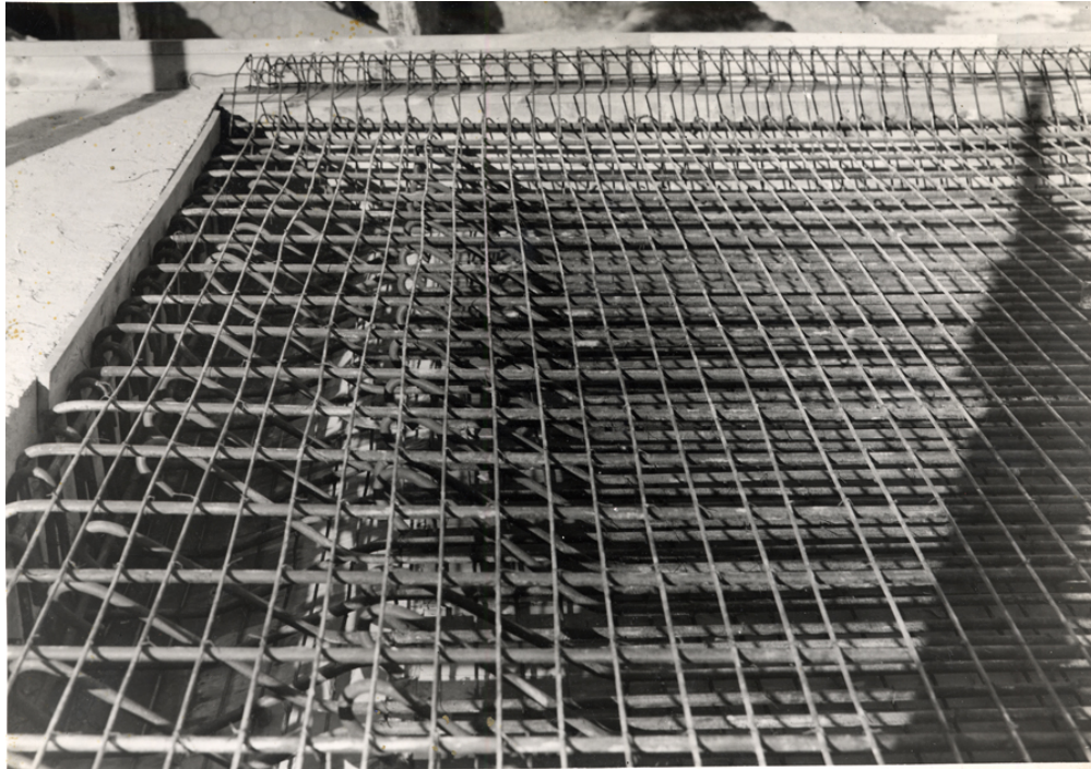
Detalle del forjado del tablero
