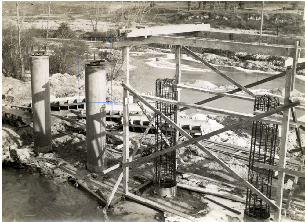
Detalle del puente en construcción
